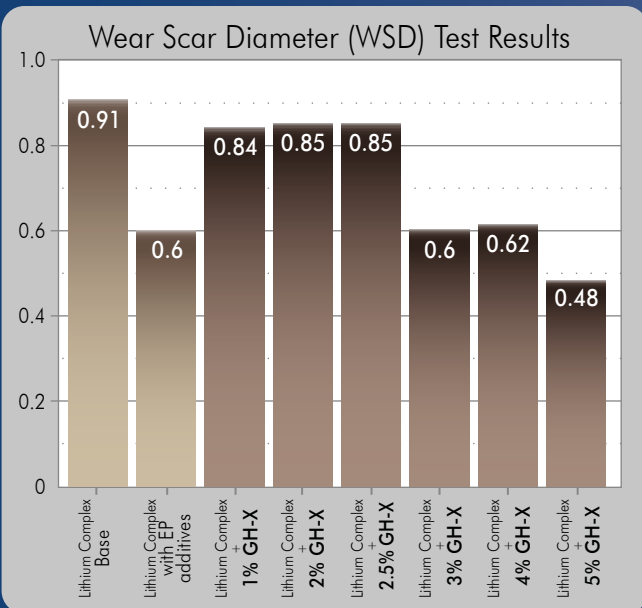
4-ball AW: ASTM D-ASTM 2266
