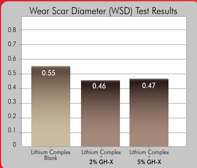
4-ball AW: ASTM D-ASTM 2266
